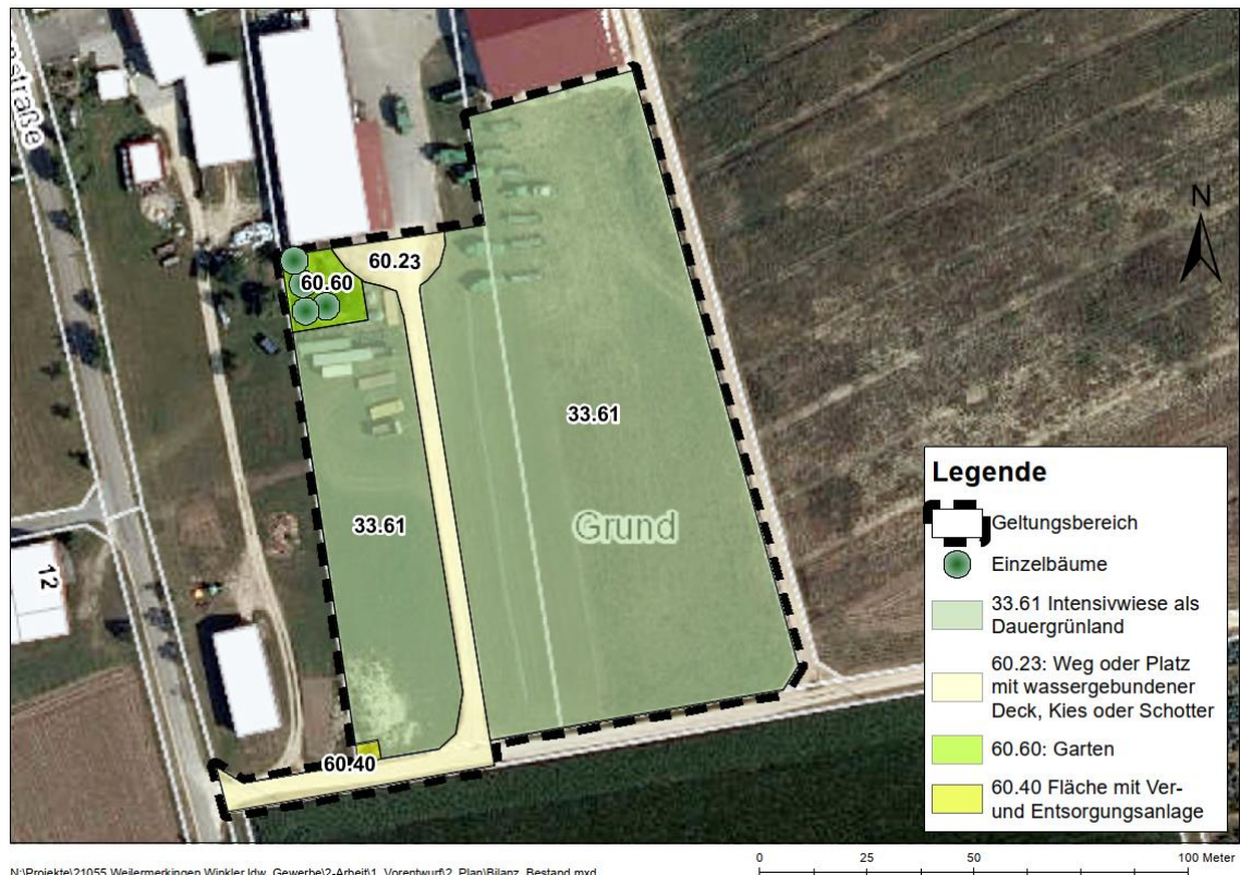
Bestandskarte der Biotoptypen im Geltungsbereich
