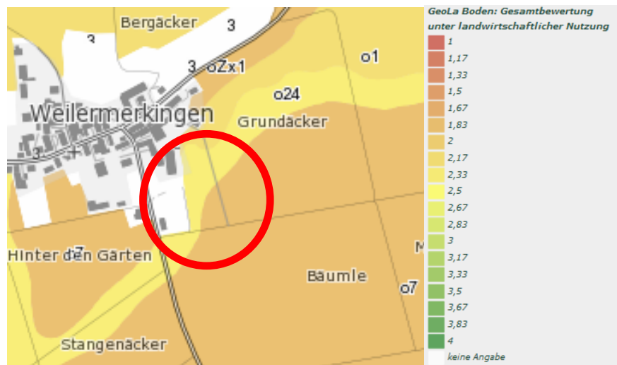
Leistungsfähigkeit (Gesamtbewertung) der Böden im Geltungsbereich (Quelle: LGRB) Geltungsbereich: rot, nördlicher Bereich (gelb hinterlegt): o24, südlicher Bereich (orange hinterlegt): Bodentyp o7.
