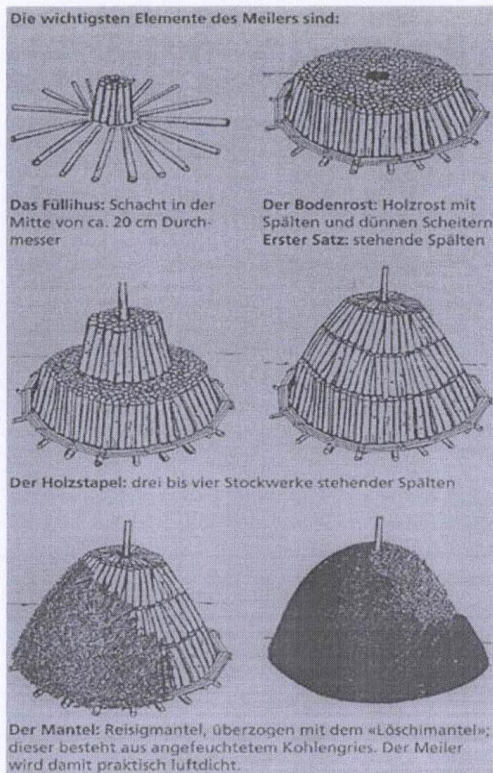
Aufbau eines Meilers
